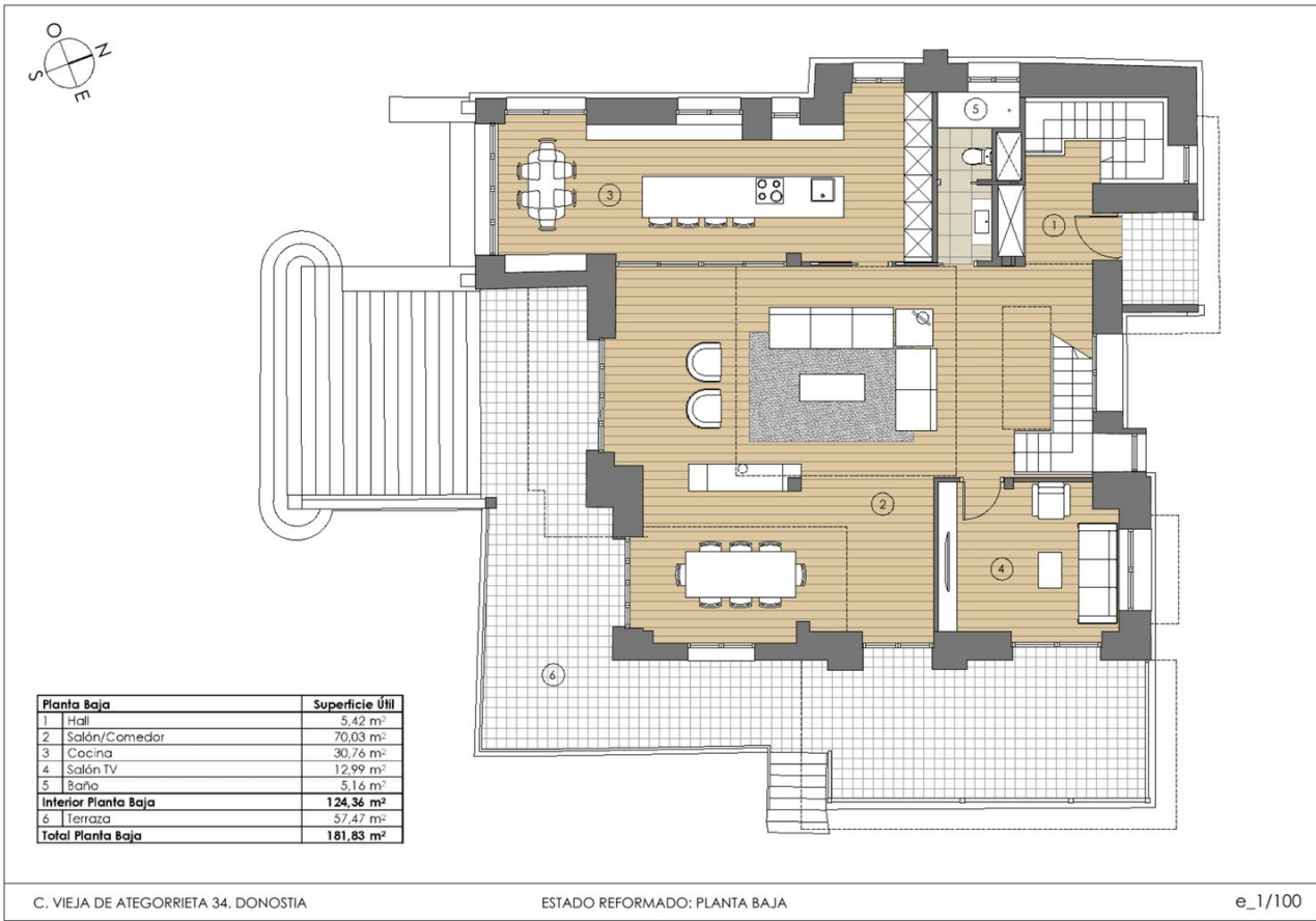
Estado reformado — planta baja. Zigor Elgoro Saldias, arquitecto. E 1/100.
